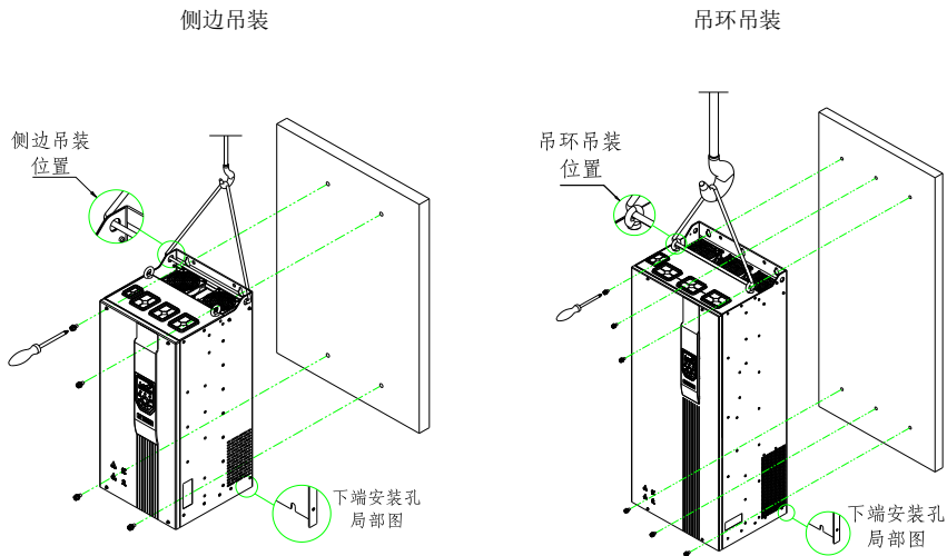
图 3-6 壁挂式安装
