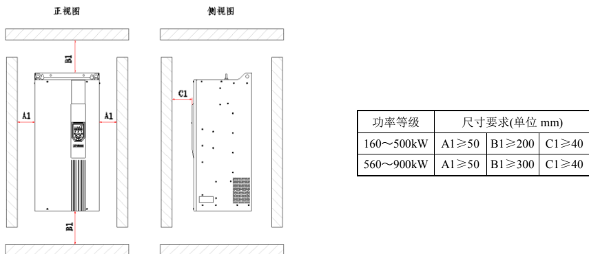
图 3-2 单台机器(Hope400S160T4~Hope400S900T4)安装间隔
