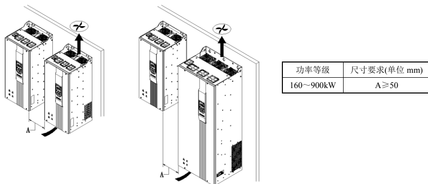
图 3-3 Hope400S160T4~Hope400S900T4 多台机器并排安装
