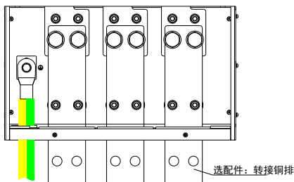
Hope400S560T4~Hope400S900T4系列软起装置 转接铜排安装示意图
