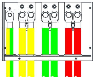
主回路端子输出端接线效果图
