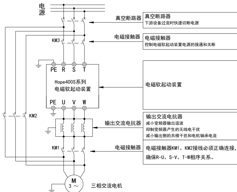
图3-9 Hope400S系列电磁软起系统连接示意图
